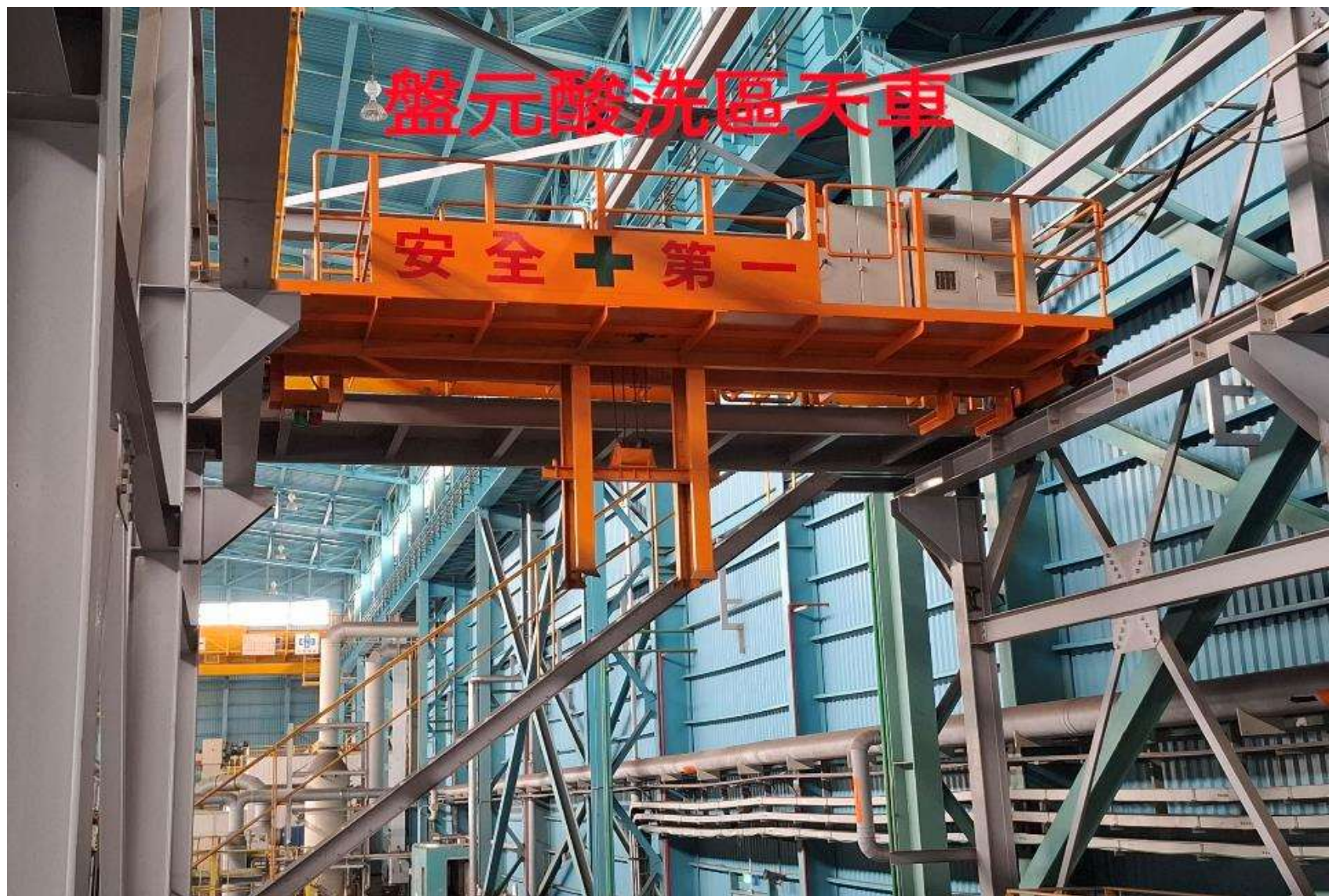
盤元酸洗區天車，資產現狀:耀一機械，積載(吊升)荷重公噸:5，普通型架空移動起重機，保留原因:拆除須搭架
