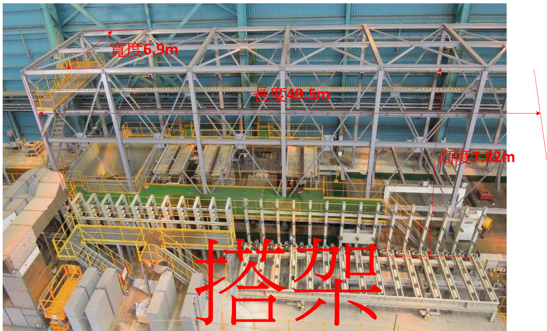
盤元酸洗區，樑柱區域長度49.5m，寬度6.9m，高度7.82m，原因:拆除須搭架
